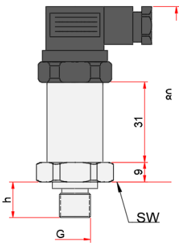
DIN 43650A
