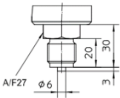
G1/2" B DIN EN 837-1
