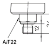
G1/2" B DIN EN ISO 1179-2
