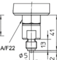
G1/4" B DIN EN 837-1
