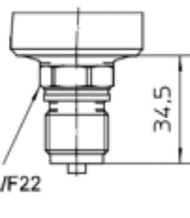
G1/2" B DIN EN 837-1 ≥ 100 bar
