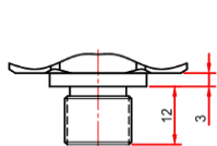
G1/4" A DIN EN ISO 1179-2
