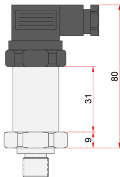
DIN 43650 A Type
