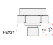
G1/4" A DIN EN ISO 1179-2
